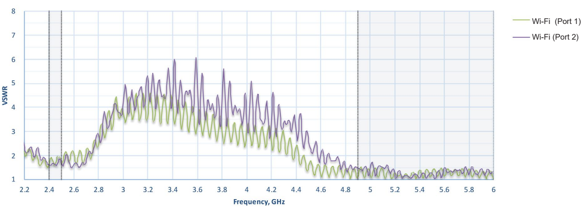
Wi-Fi Antenna VSMR
